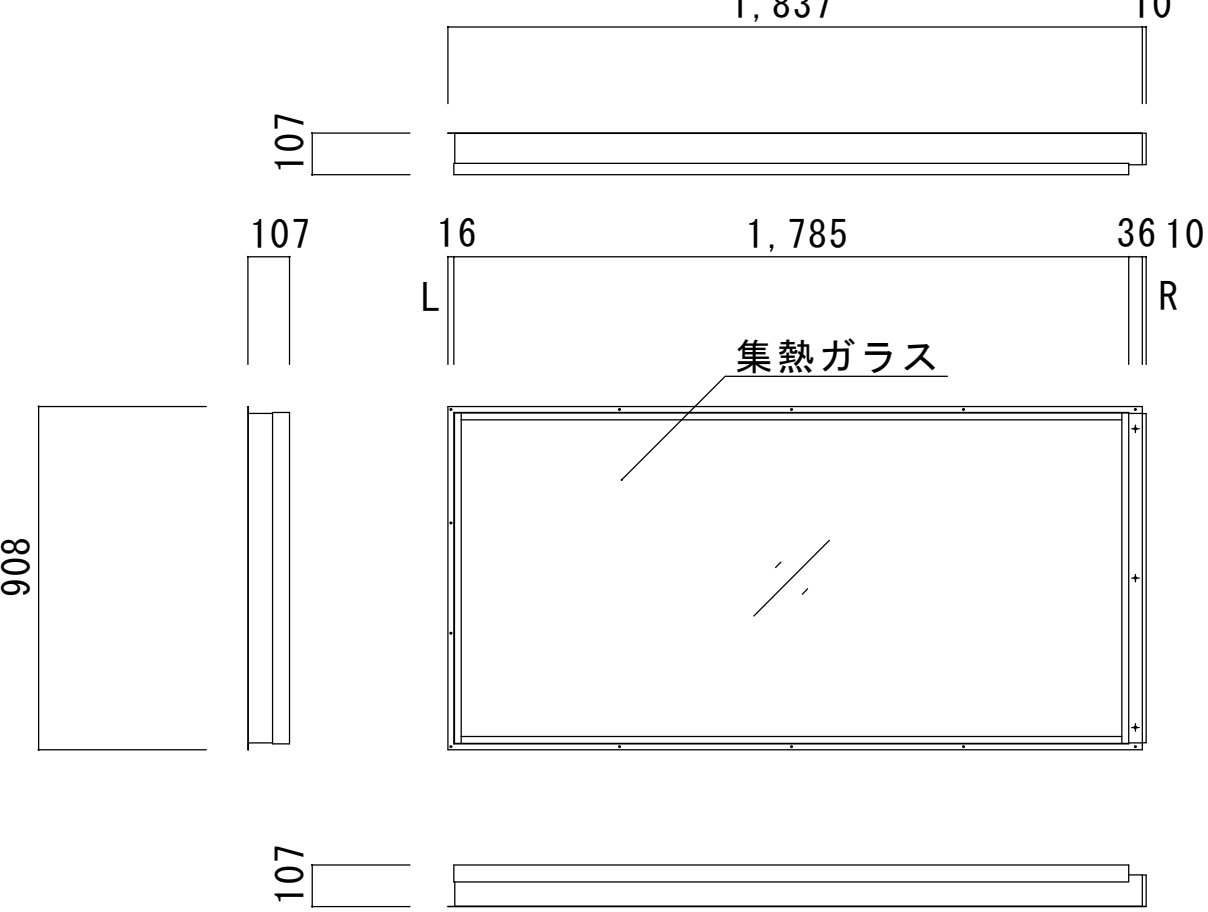
横設置型集熱パネル・L仕様
