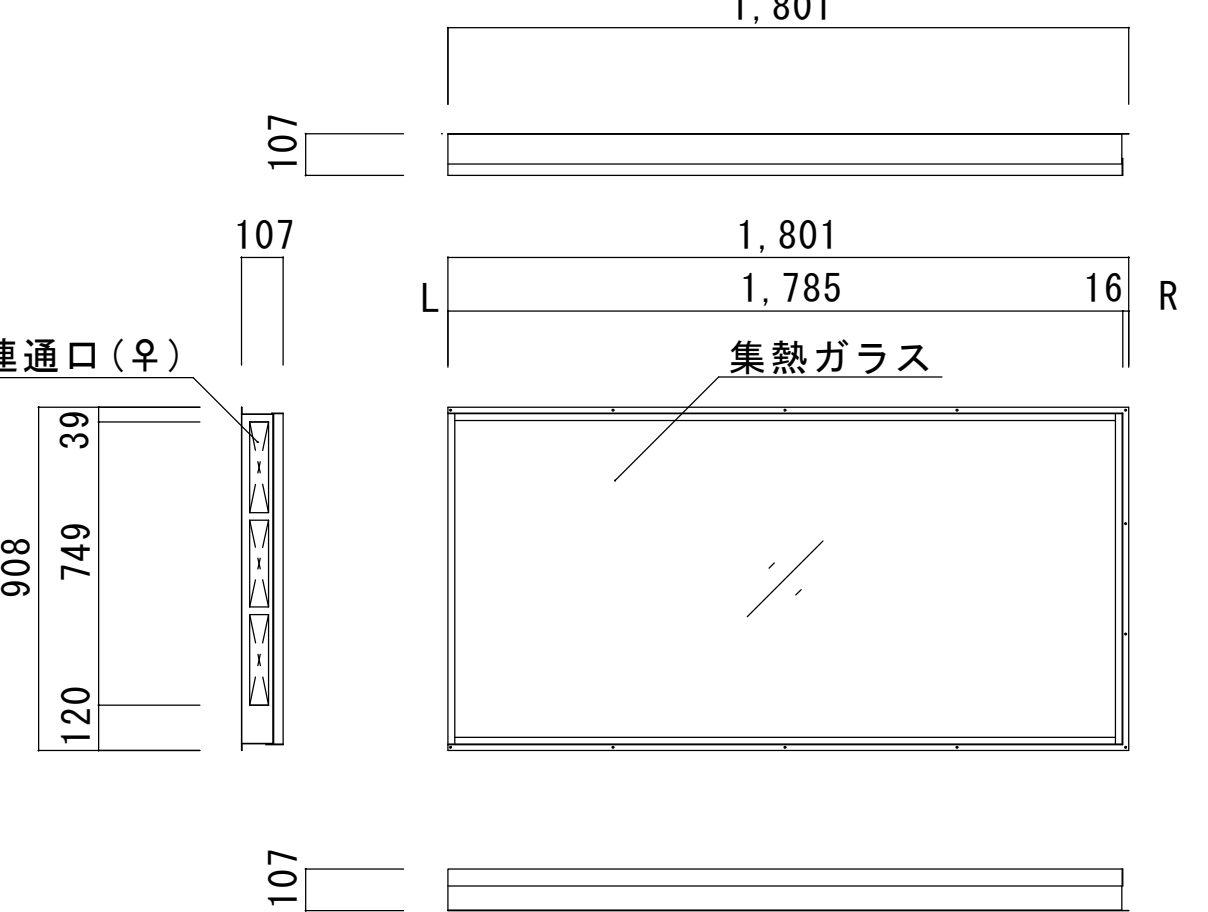
横設置型集熱パネル・R仕様
