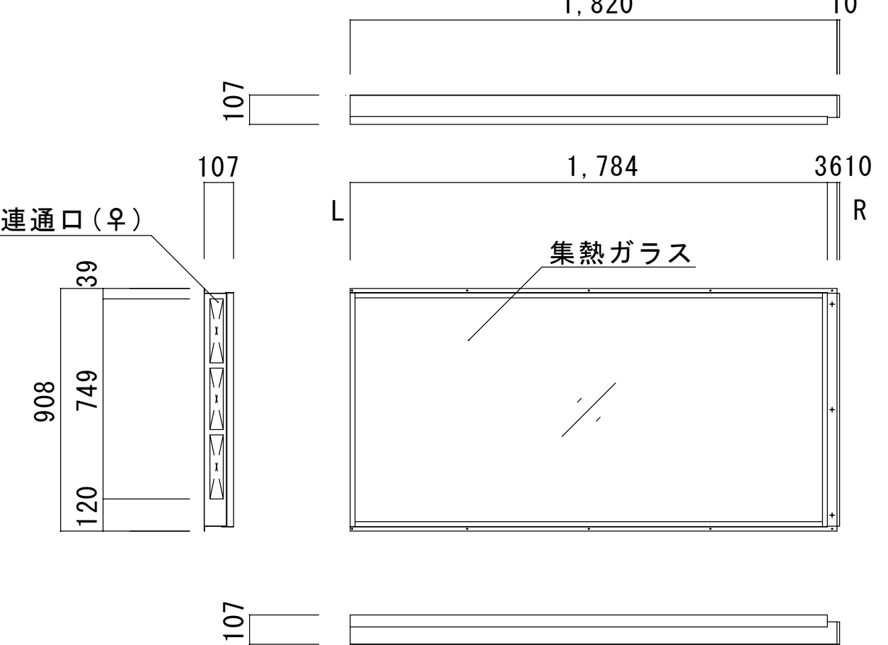
横設置型集熱パネル・C仕様
