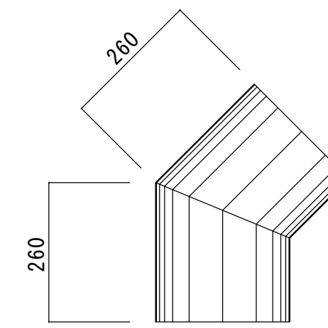
45° エルボ
