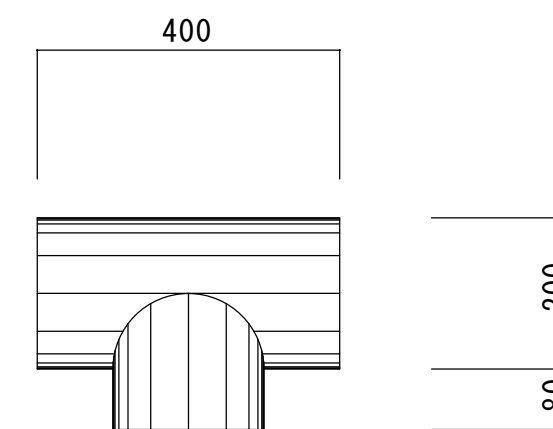
TEE
