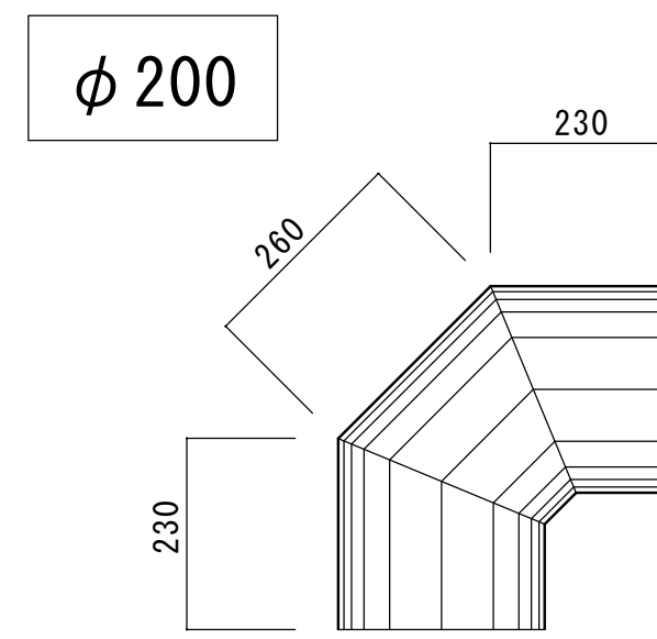
90° エルボ
