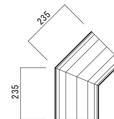
45° エルボ
