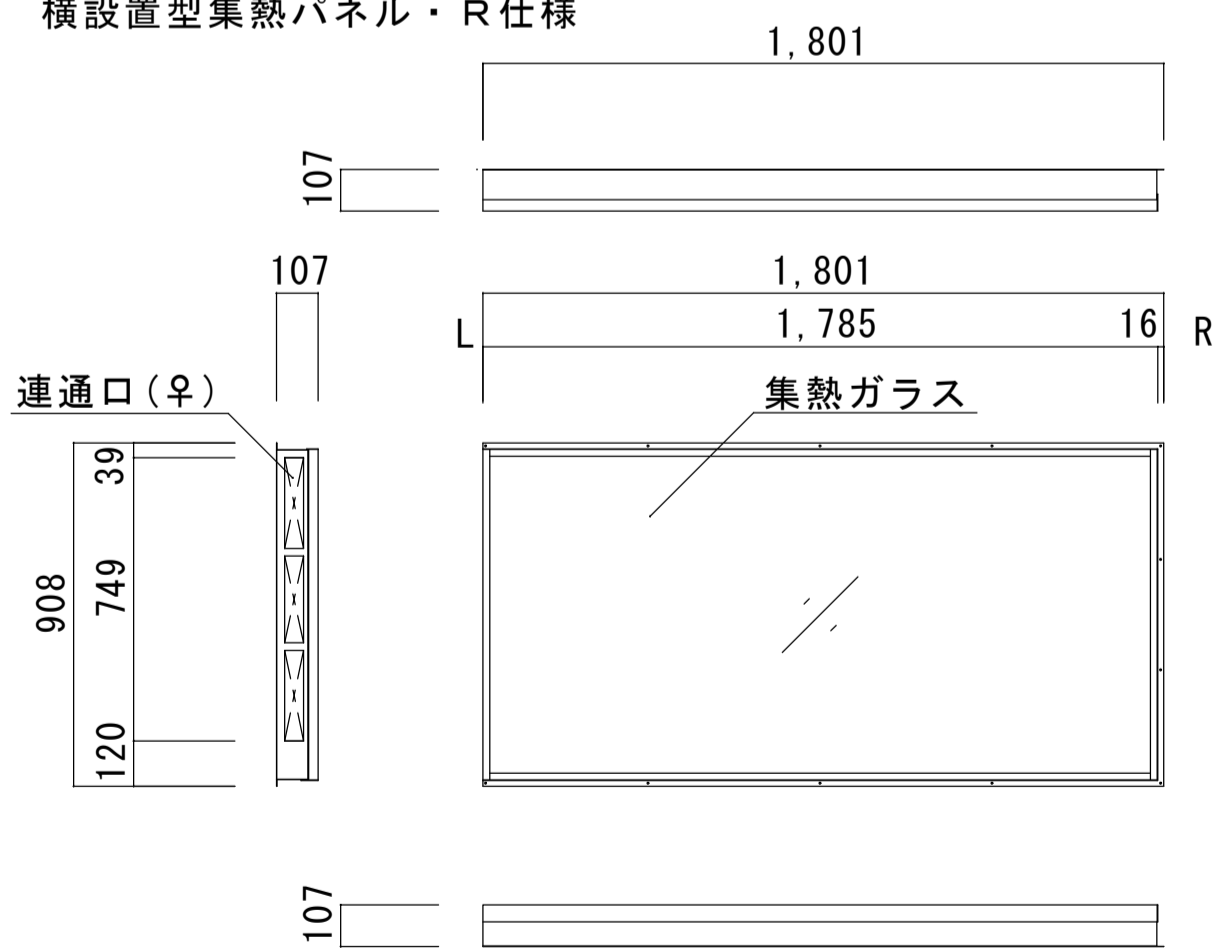
横設置型集熱パネル・R仕様
