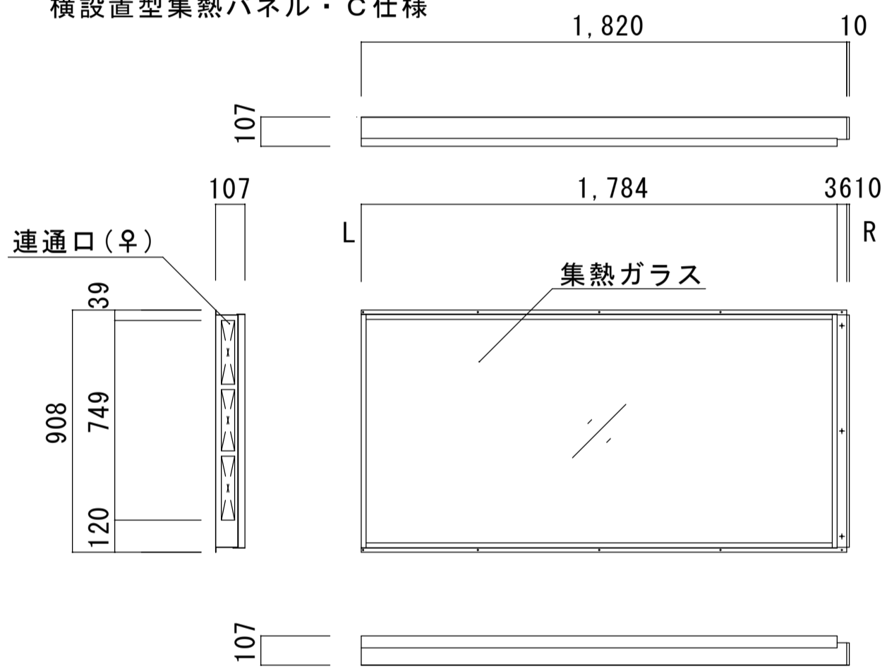
横設置型集熱パネル・C仕様
