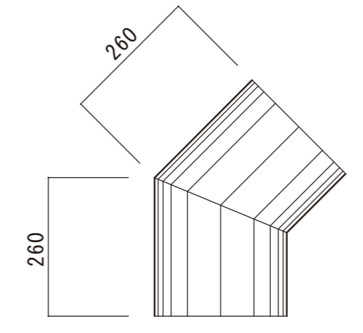
45° エルボ
