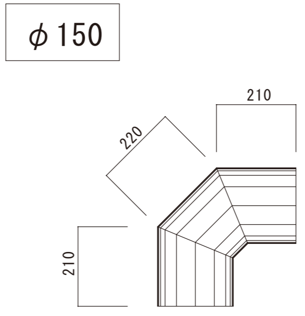
90° エルボ
