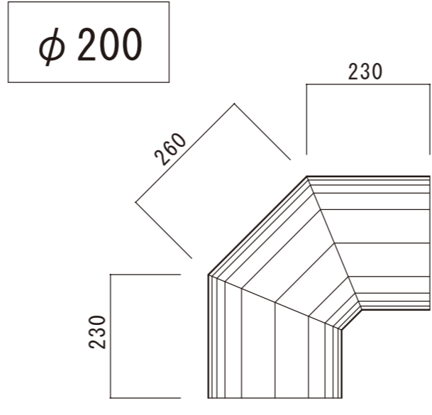
90° エルボ
