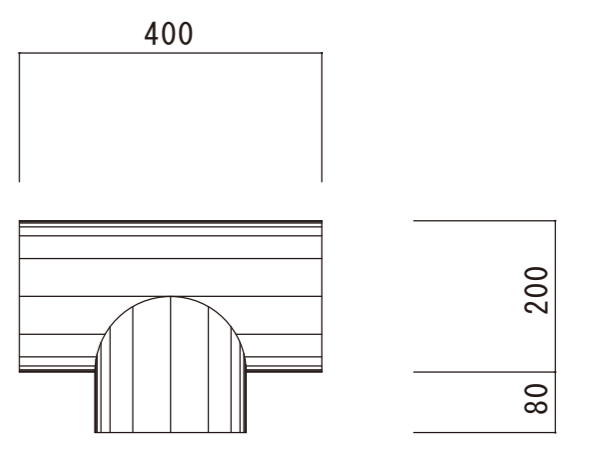
TEE
