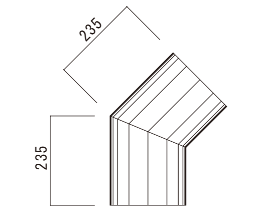
45° エルボ
